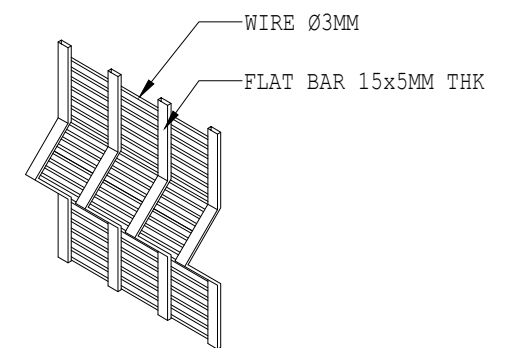
ISOMETRIC Scale: NTS
