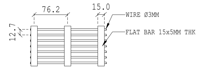
3 DETAIL Scale: NTS
